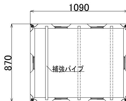
水洗架台平面図
