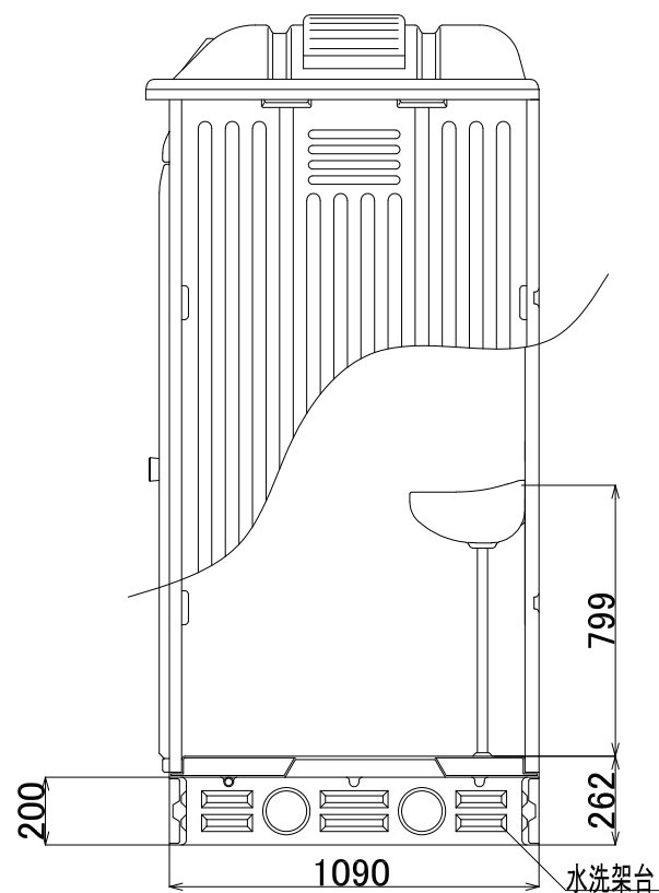
側面及び部分断面図
