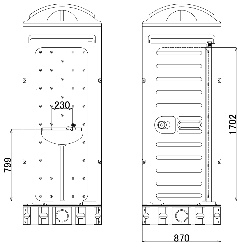
正面図
