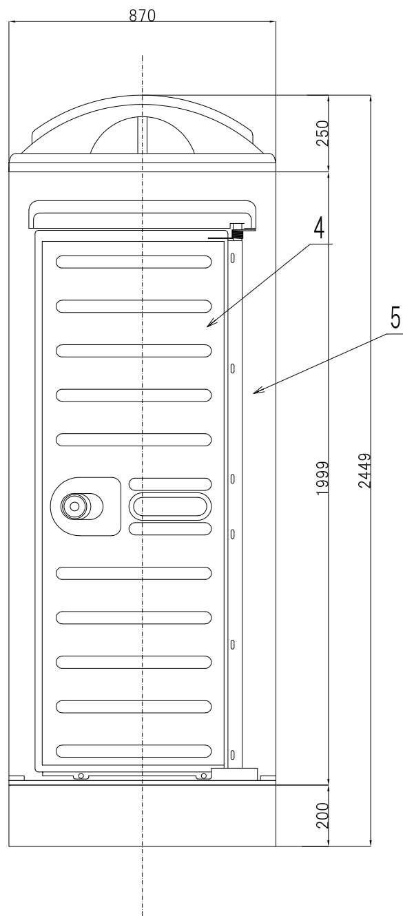
正面図
